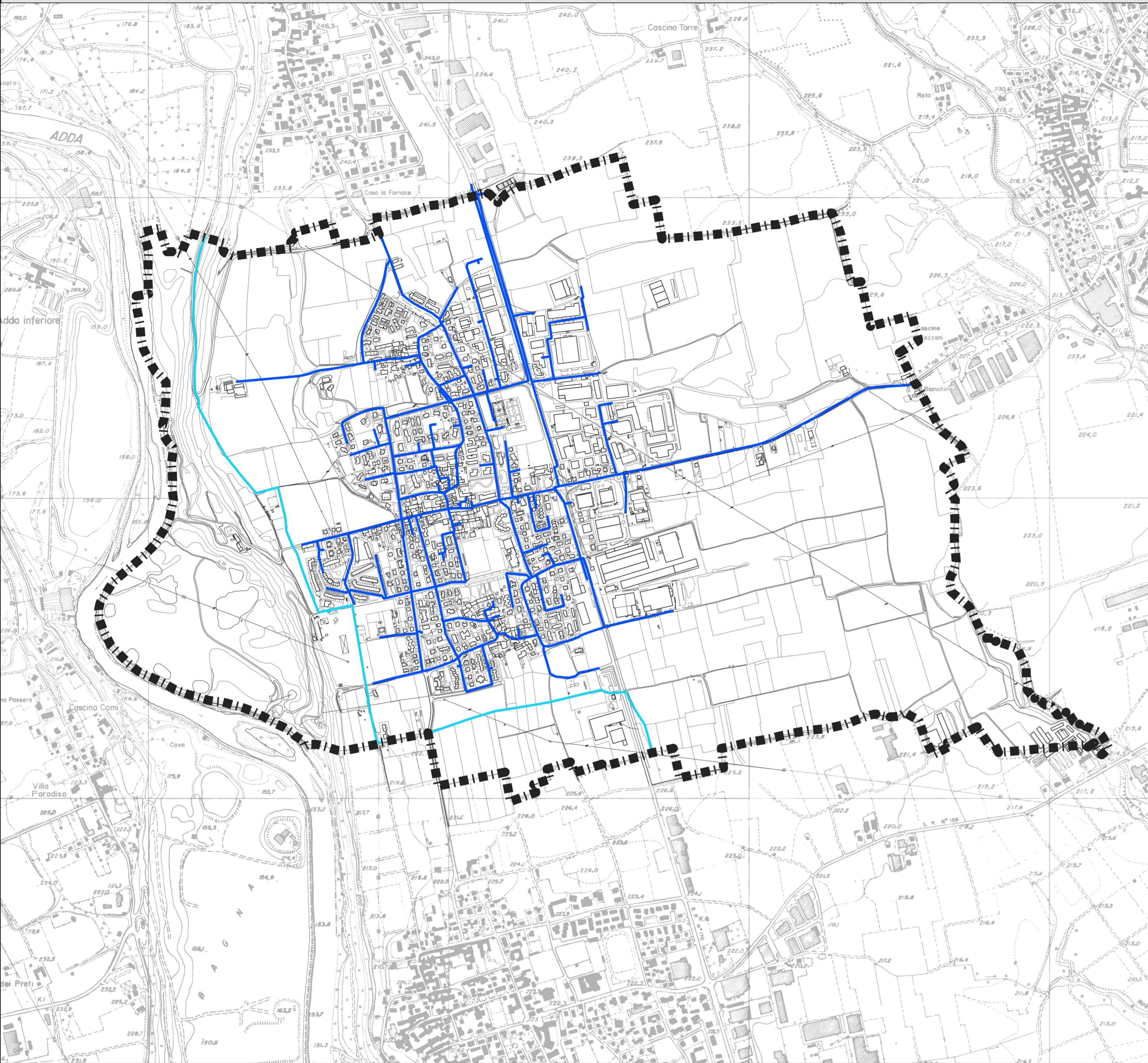
RETE ACQUEDOTTO
