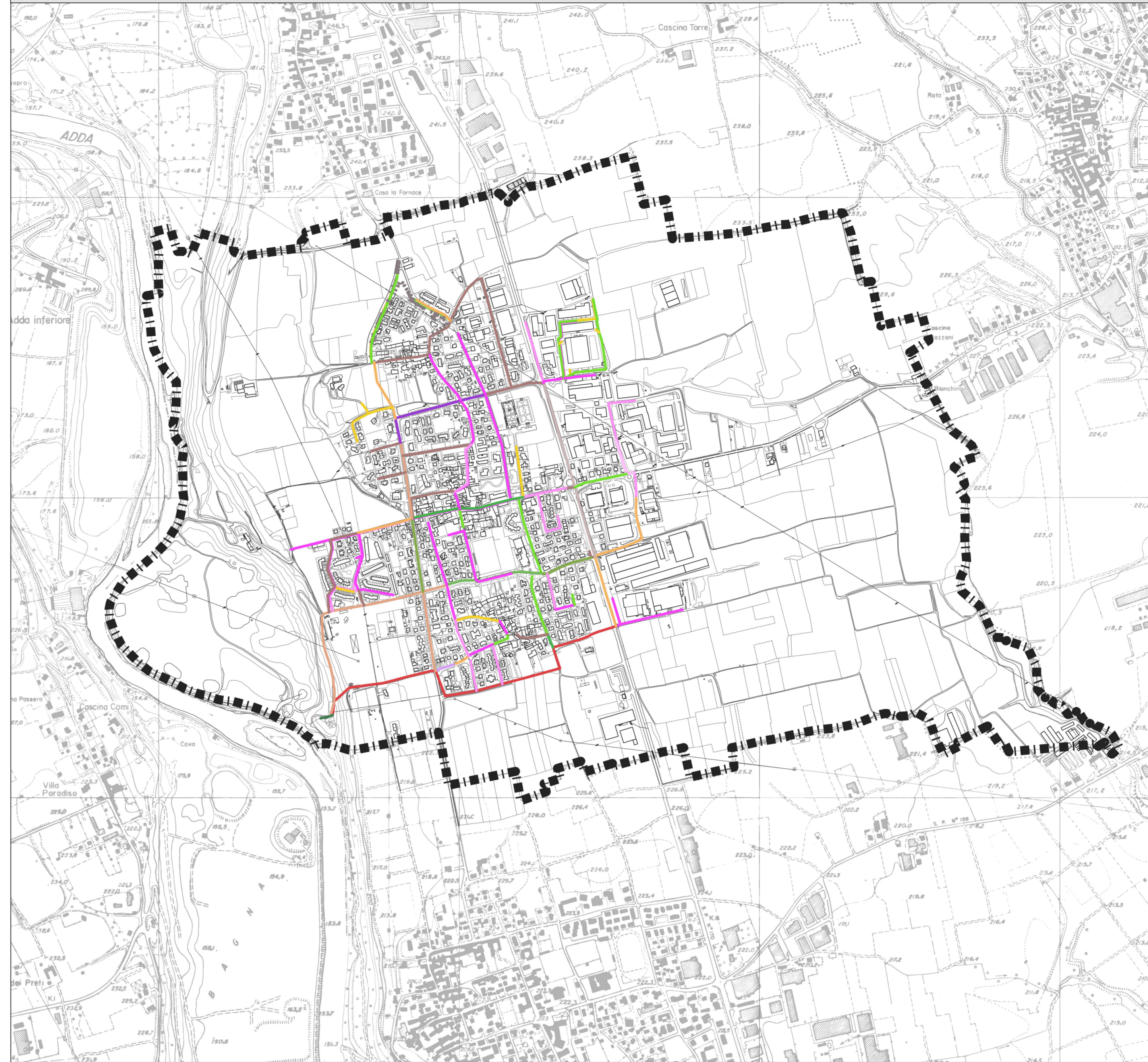
RETE FOGNARIA
