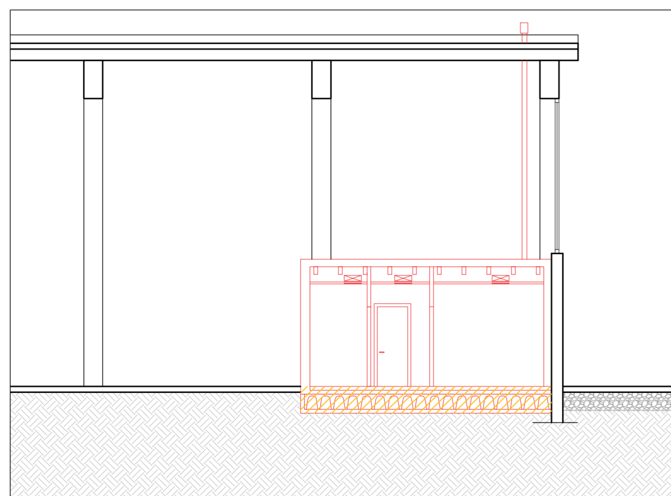
SEZIONE CONFRONTO
