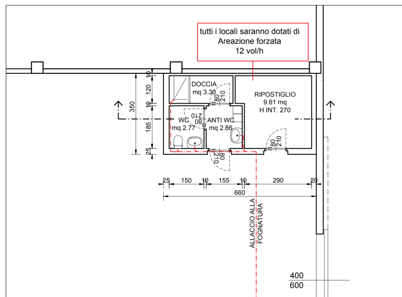
PIANTA PROGETTO
