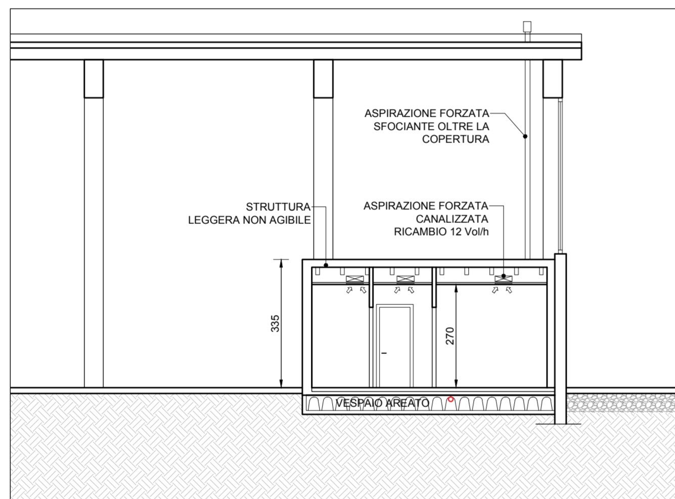
SEZIONE PROGETTO
