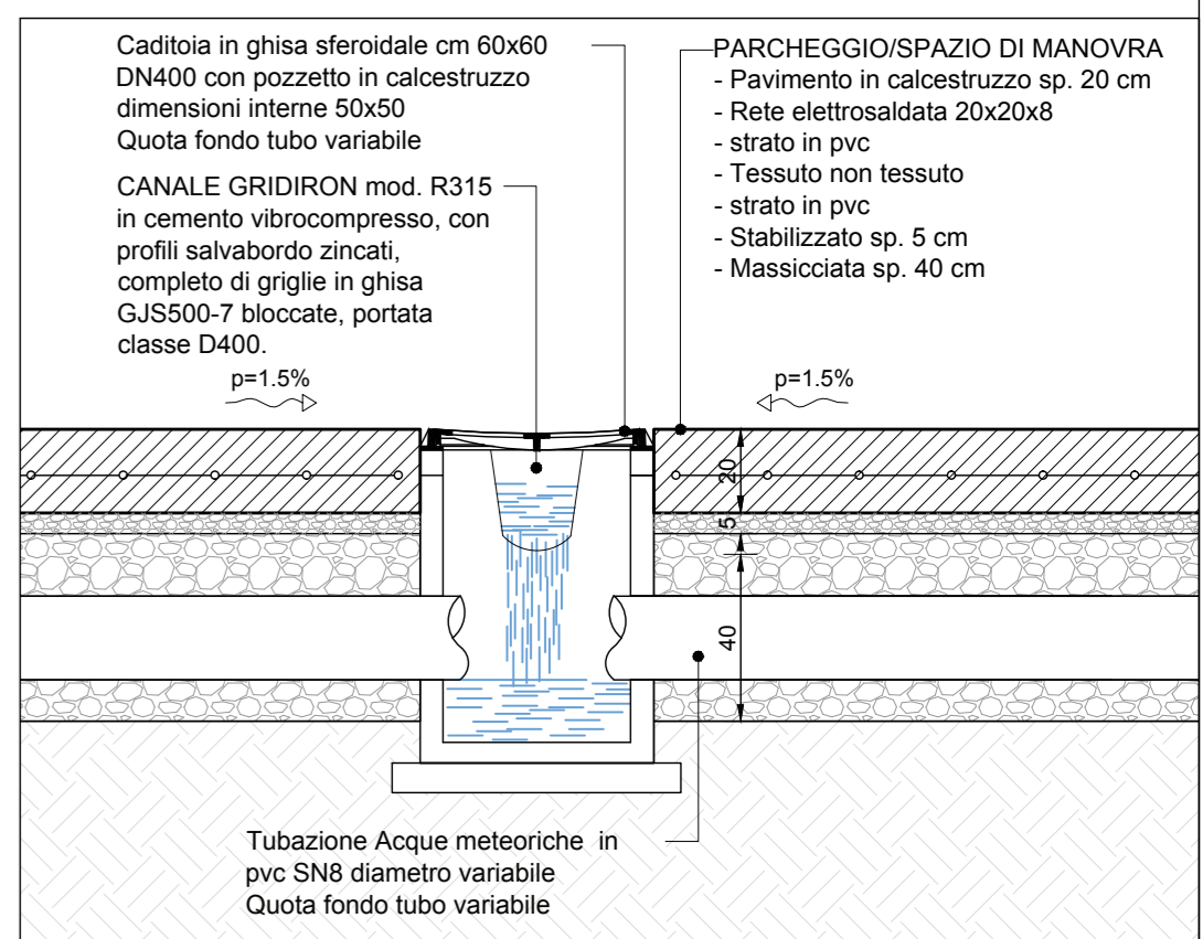
DETTAGLIO PAVIMENTAZIONE E RACCOLTA ACQUE METEORICHE scala 1:20
