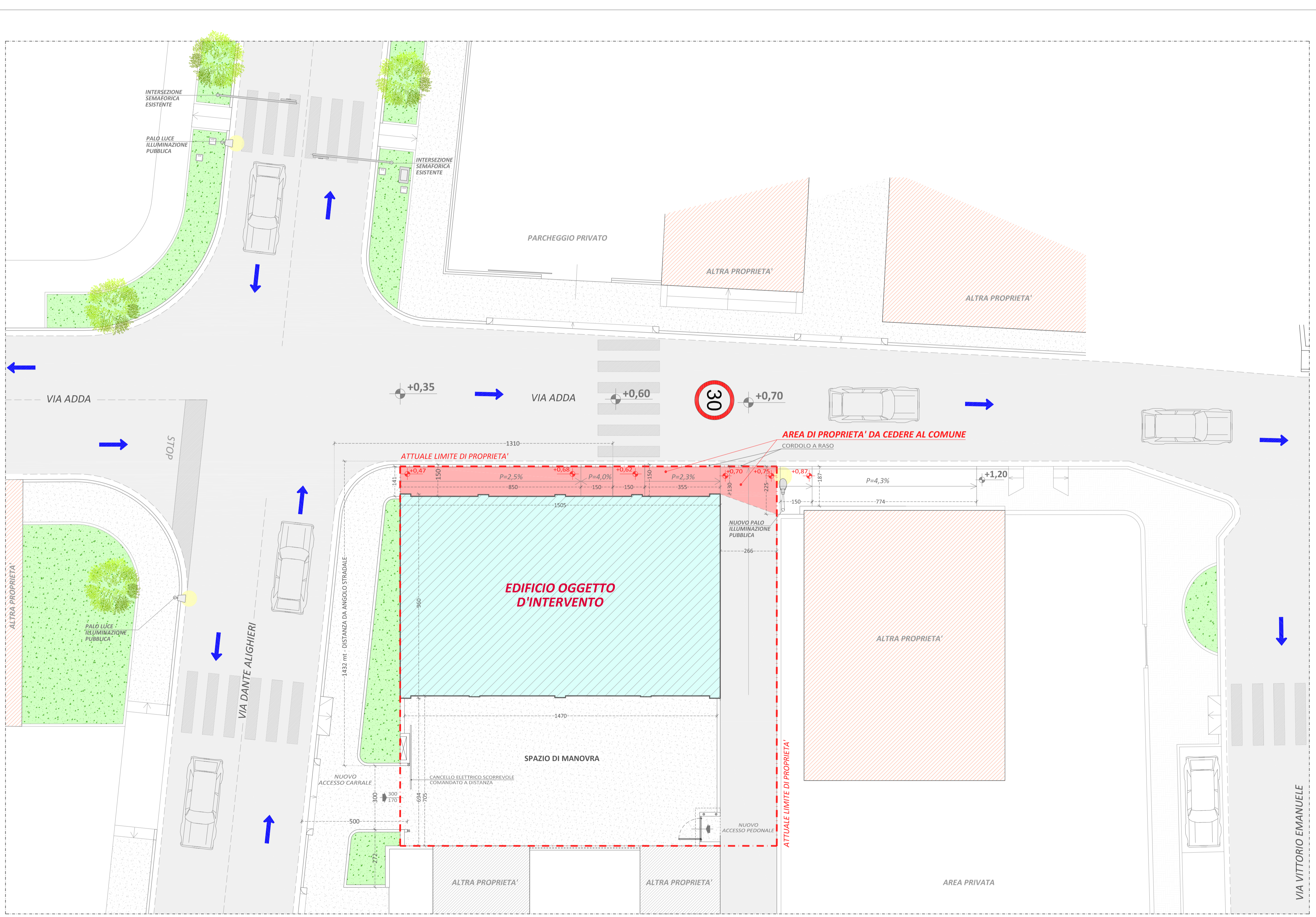
STRALCIO PLANIMETRICO
