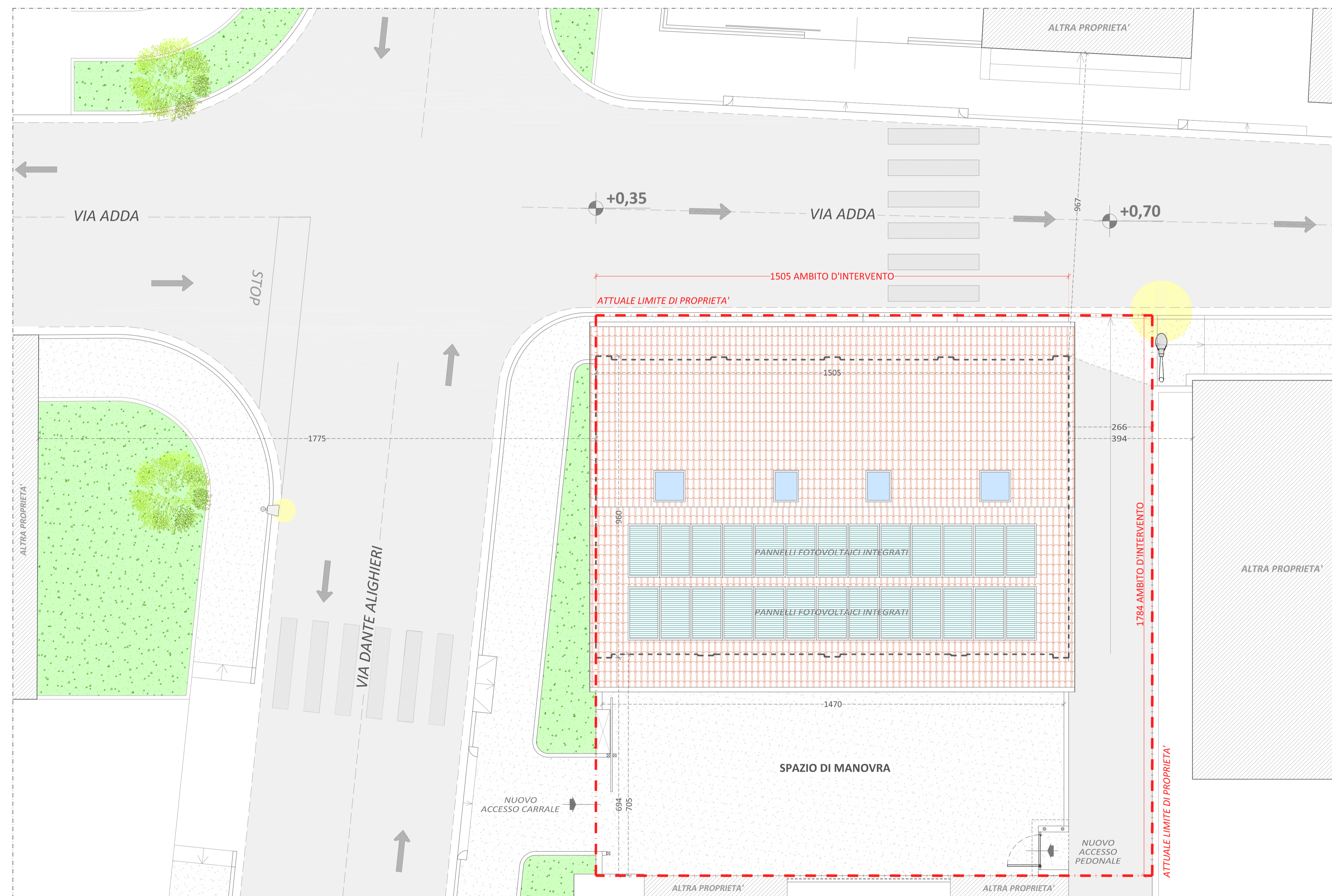
STRALCIO PLANIMETRICO
